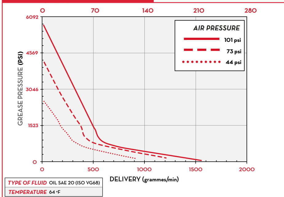
PIUSI P60:1 - 470
